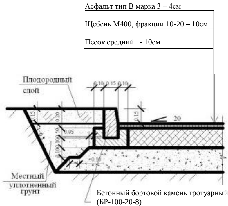
Рисунок 24. Слои асфальтового покрытия
