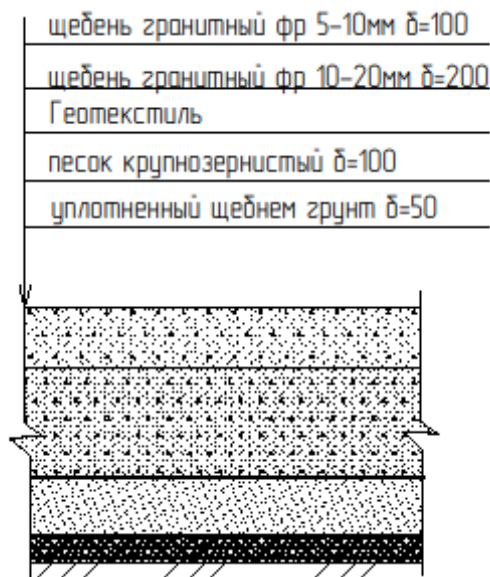
Рисунок 10. Слои щебеночно-гравийного покрытия
