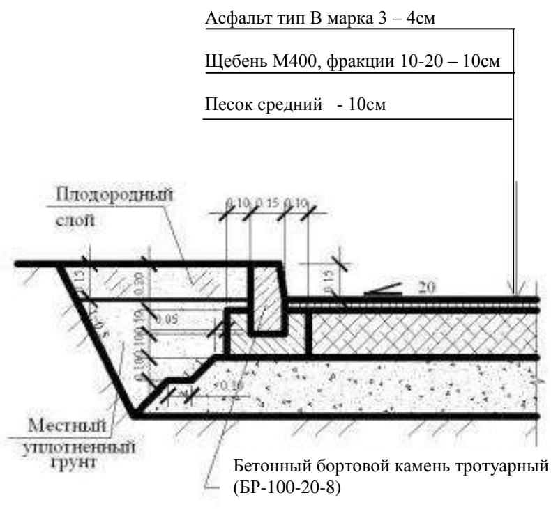
Рисунок 5. Слои асфальтового покрытия
